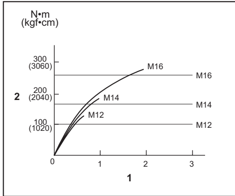
1. Kinnitamisae (sekund) 2. Väändemoment
