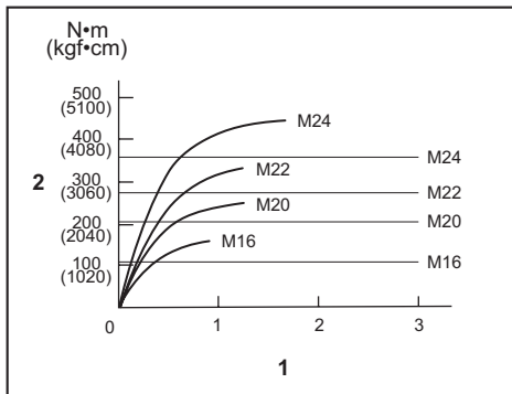
1. Pievilksanas laiks (sekundēs) 2. Pievilksanas griezes moments
