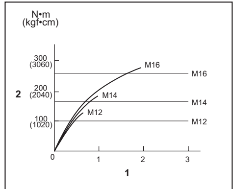
1. Pievilksanas laiks (sekundēs) 2. Pievilksanas griezes moments
